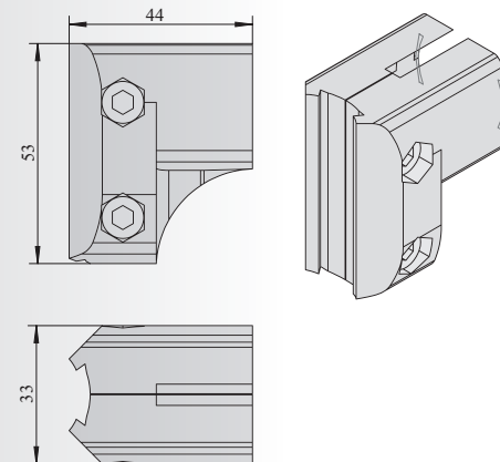
加强外直接头 Strengthen Connector Outer Type
