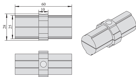
基础线棒延伸接头 Direct Extending Connector
