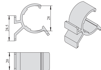
标牌卡扣 Signboard Clip
