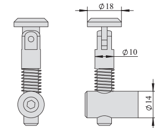
4545 转角 90° 型 LS-4545 Oblique 90-Degree Type
