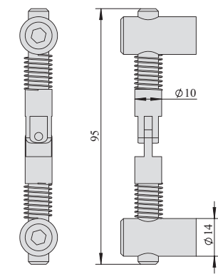
4545 对角 90° 型 LS-4545 Miter 90-Degree Type
