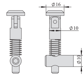
4040 转角 0° 型 LS-4040 Oblique 0-Degree Type
