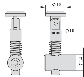
4545 转角 0° 型 LS-4545 Oblique 0-Degree Type
