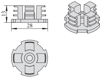
加强线棒堵头 Loaded Frame Insert
