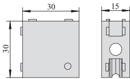
1530 下滑块 1530 Lower slider
