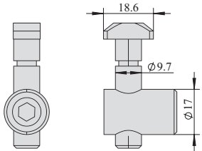
4545 直角 0° 型 4545 Right-angle 0-Degree Type
