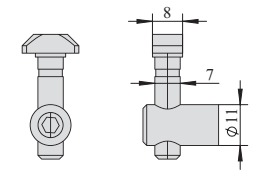
3040 直角 90° 型 LS-30 & LS-40 Right-angle 90-Degree Type
