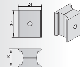
平行固定接头 B-L30 Parallel Fixed Connector B-L30
