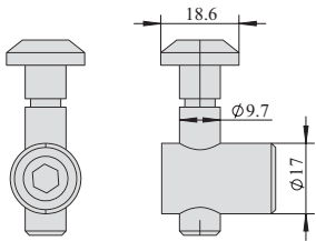
4545 直角万向型 LS-4545 90-Degree Universal Type
