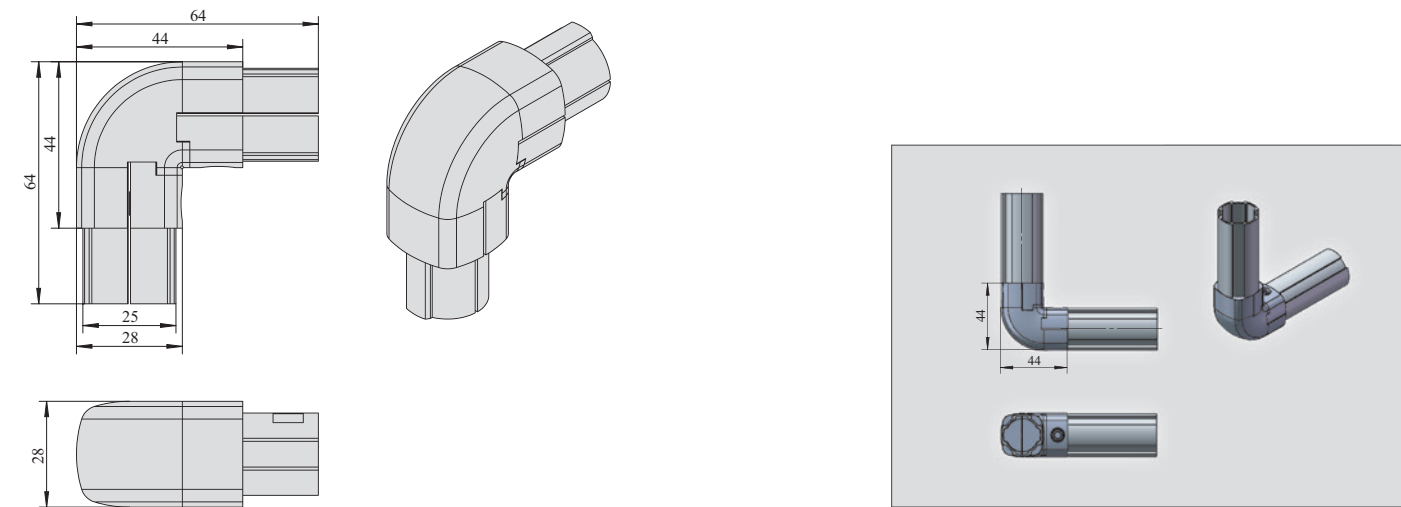
90° 内接头 Connector Inner Type 90°
