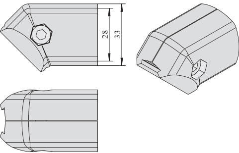
45° 外接头 Connector Outer Type 45°
