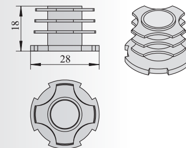
基础线棒堵头 Inner Cap
