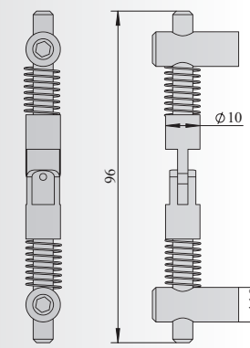
4040 对角 90° 型 LS-4040 Miter 90-Degree Type
