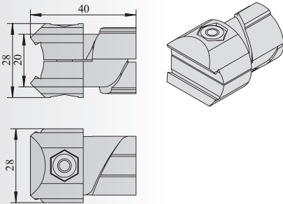
内直接头 Connector Inner Type
