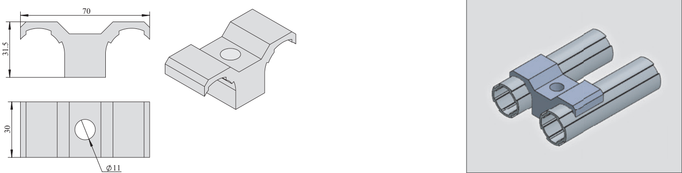
脚轮固定组件 Caster Supportor
