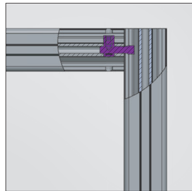
4545 直角 90° 型 LS-4545 Right-angle 90-Degree Type
