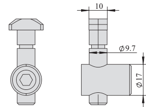
4545 直角 90° 型 LS-4545 Right-angle 90-Degree Type
