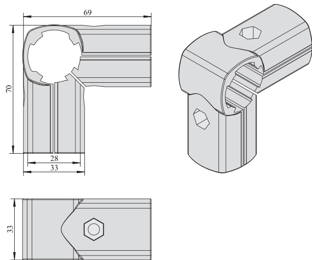
外抱 90° 接头 Connector Vertical Type 90°
