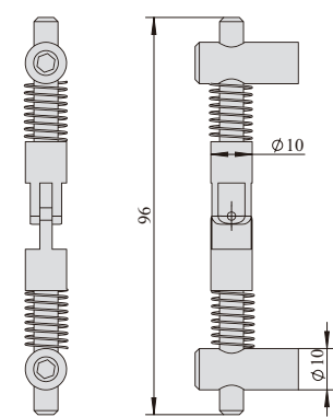
4040 对角 0° 型 LS-4040 Miter 0-Degree Type
