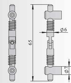
2020 对角 90° 型 LS-2020 Miter 90-Degree Type
