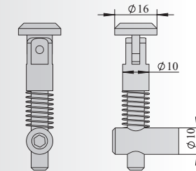
4040 转角 90° 型 LS-4040 Oblique 90-Degree Type
