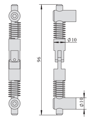
3030 对角 90° 型 LS-3030 Miter 90-Degree Type
