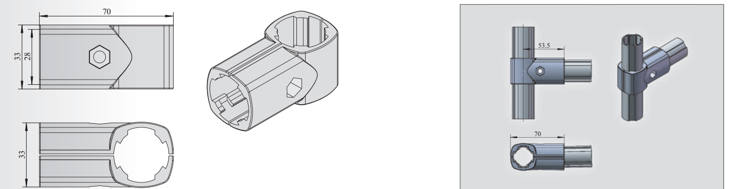
外抱直接头 Connector Vertical Type
