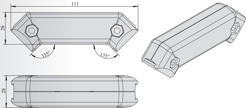
45° 加强接头 Strengthen Connector 45°
