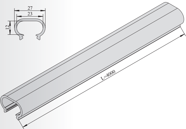
暗藏式导线卡槽 Hidden Wire Slot
