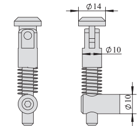
3030 转角 90° 型 LS-3030 Oblique 90-Degree Type
