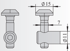
3040 直角万向型 LS-30 & LS-40 90-Degree Universal Type
