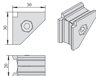
90° 直角固定接头 Fixed Connector 90°
