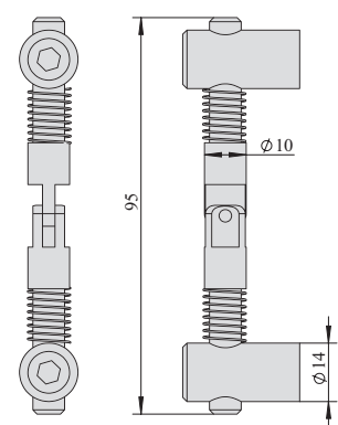
4545 对角 0° 型 LS-4545 Miter 0-Degree Type
