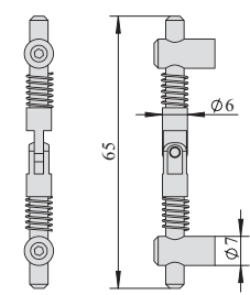
2020 对角 0° 型 LS-2020 Miter 0-Degree Type
