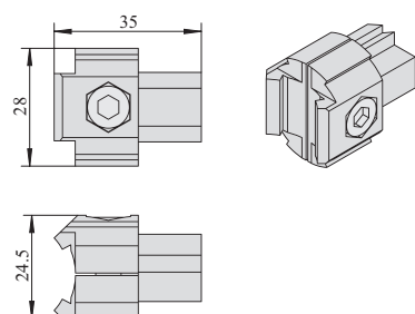
T 型槽内直接头 T-groove Connector
