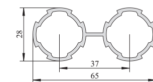
双联基础线棒 Duplex Foundation Frame
