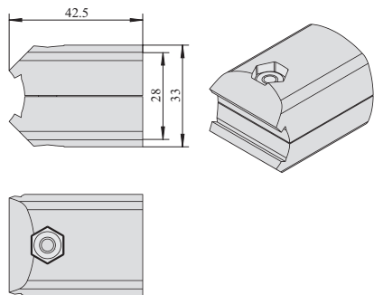
外直接头 Multi Connector Outer Type
