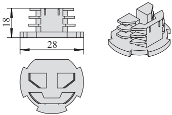
T 型槽线棒堵头 T Slot Frame Insert
