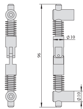
3030 对角 0° 型 LS-3030 Miter 0-Degree Type
