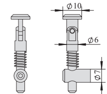
2020 转角 0° 型 LS-2020 Oblique 0-Degree Type
