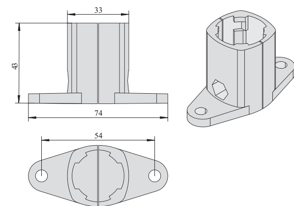
外抱式底座 External Holding Pedestal
