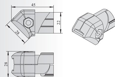
45° 内接头 Connector Inner Type 45°
